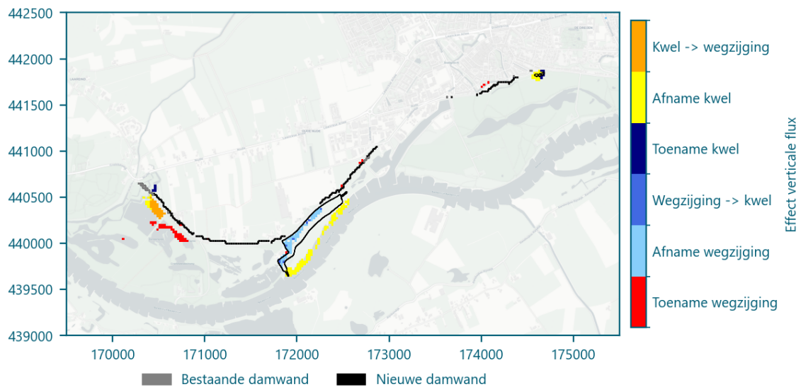
Afbeelding III.4 Verandering van de verticale flux in april 2017 na de dijkversterking en de natuuropgaven in ontwerploop 2
