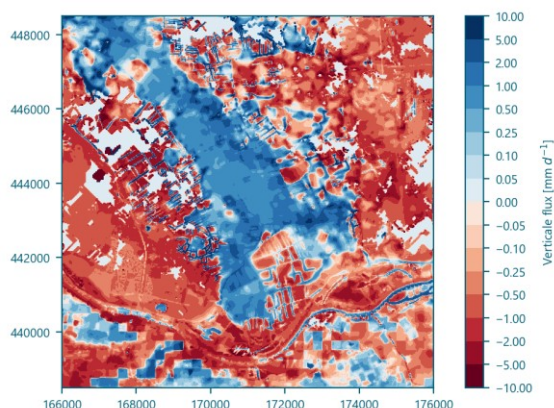
Afbeelding 4.6 Verticale flux van de Gemiddeld Hoogste Grondwaterstand (GHG) van 2009-2017 (mm/d) in de referentiesituatie
