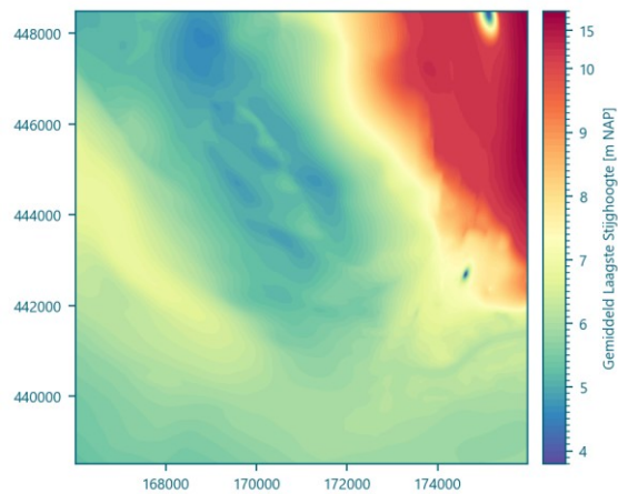
Afbeelding II.5 Gemiddeld Laagste Stijghoogte (GLS) referentiesituatie in modellaag 3
