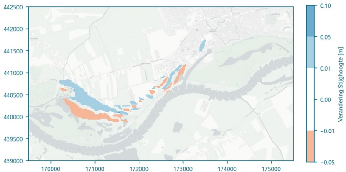
Afbeelding 3.6 Verandering van de Gemiddeld Hoogste Stijghoogte (GHS) van de 2 e modellaag van 2009-2017 volgens uit de aangepaste horizontale anisotropie
