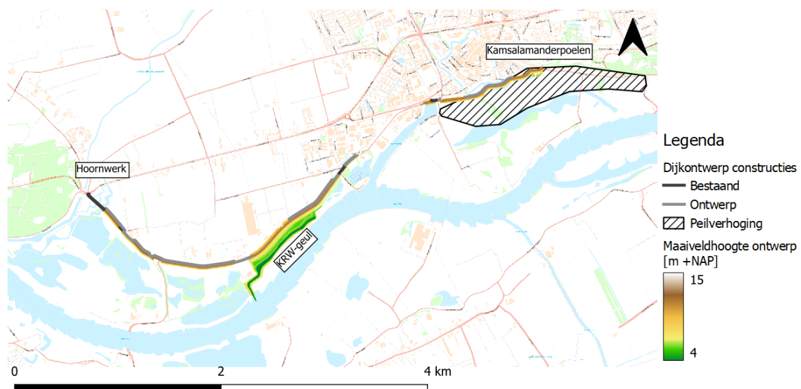
Afbeelding 3.1 Overzicht van de dijkversterking en de natuuropgaven van de Grebbedijk in ontwerploop 2
