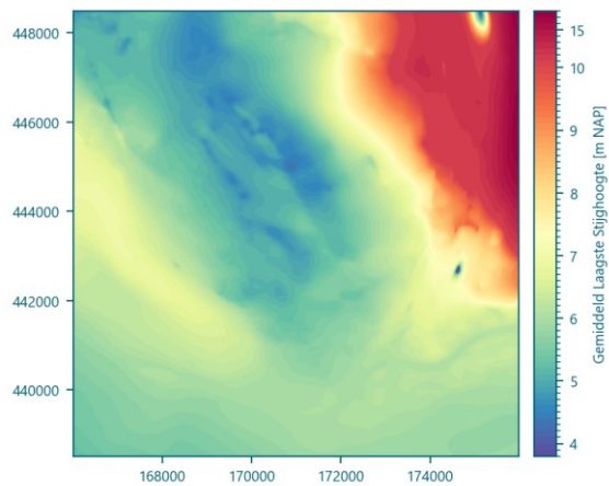
Afbeelding II.1 Gemiddeld Laagste Stijghoogte (GLS) referentiesituatie in modellaag 2
