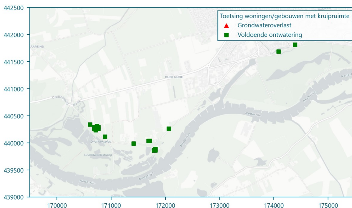
Afbeelding 4.14 Toetsing ontwatering van woningen/gebouwen met kruipruimte met een ontwateringsdiepte van 0,7 m bij de Gemiddeld Hoogste Grondwaterstand (GHG) van 2009-2017 van ontwerploop 2
