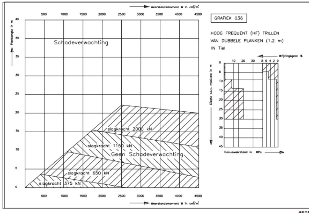
Afbeelding III.3 NVAF/PSD-grafiek voor hoog frequent trillen van dubbele damwandplanken in Tiel volgens de CUR166 [ref. 3]
