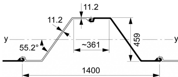
Afbeelding 2.4 Afmetingen dubbele damwand type AZ24-700 (ref. 2)
