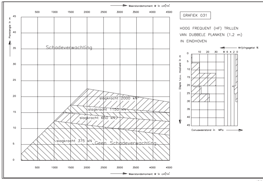
Afbeelding III.4 NVAF/PSD-grafiek voor hoog frequent trillen van dubbele damwandplanken in Eindhoven volgens de CUR166 [ref. 3]
