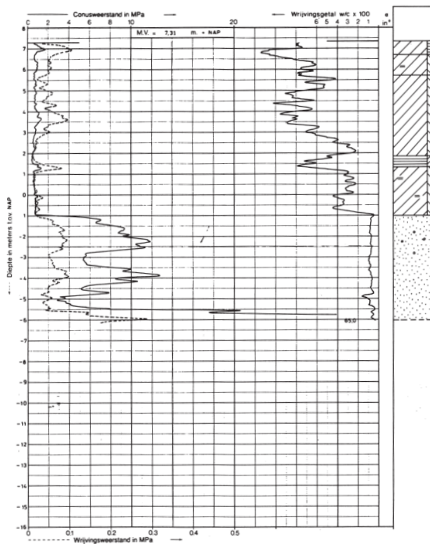
Afbeelding III.1 Sondering Tiel volgens de CUR166 [ref. 3]
